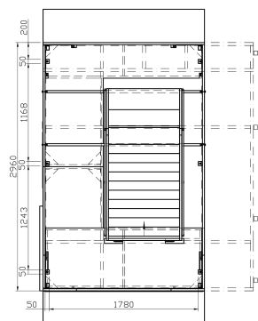
A-A M 1:1
