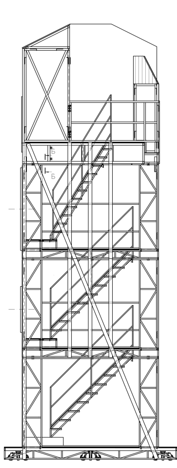
A-A M 1:1
