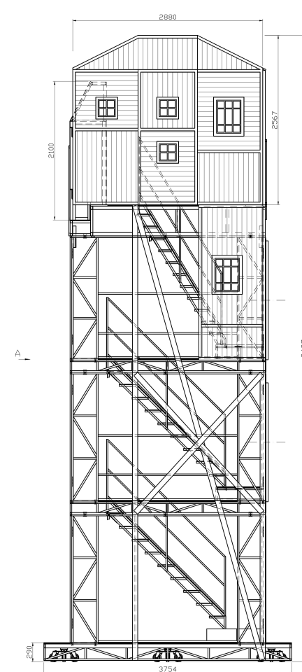
B-B M 1:1
