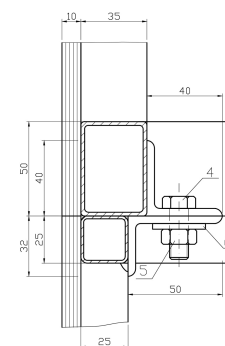
B-B M 1:1
